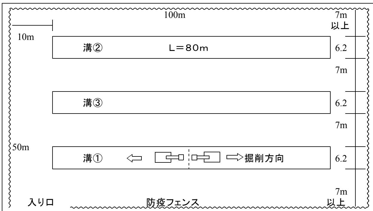
【平面図】
