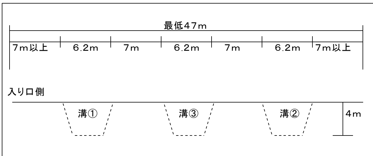
【断面図】
