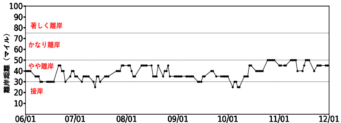
図1 都井岬沖の黒潮流軸の離岸距離（海上保安庁海洋情報部 HP よりデータ取得）
