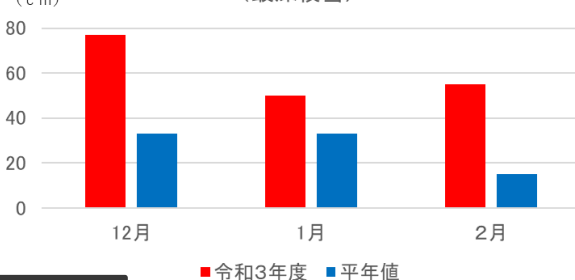
令和3年12月25日からの大雪と平年値との比較 (最深積雪)
